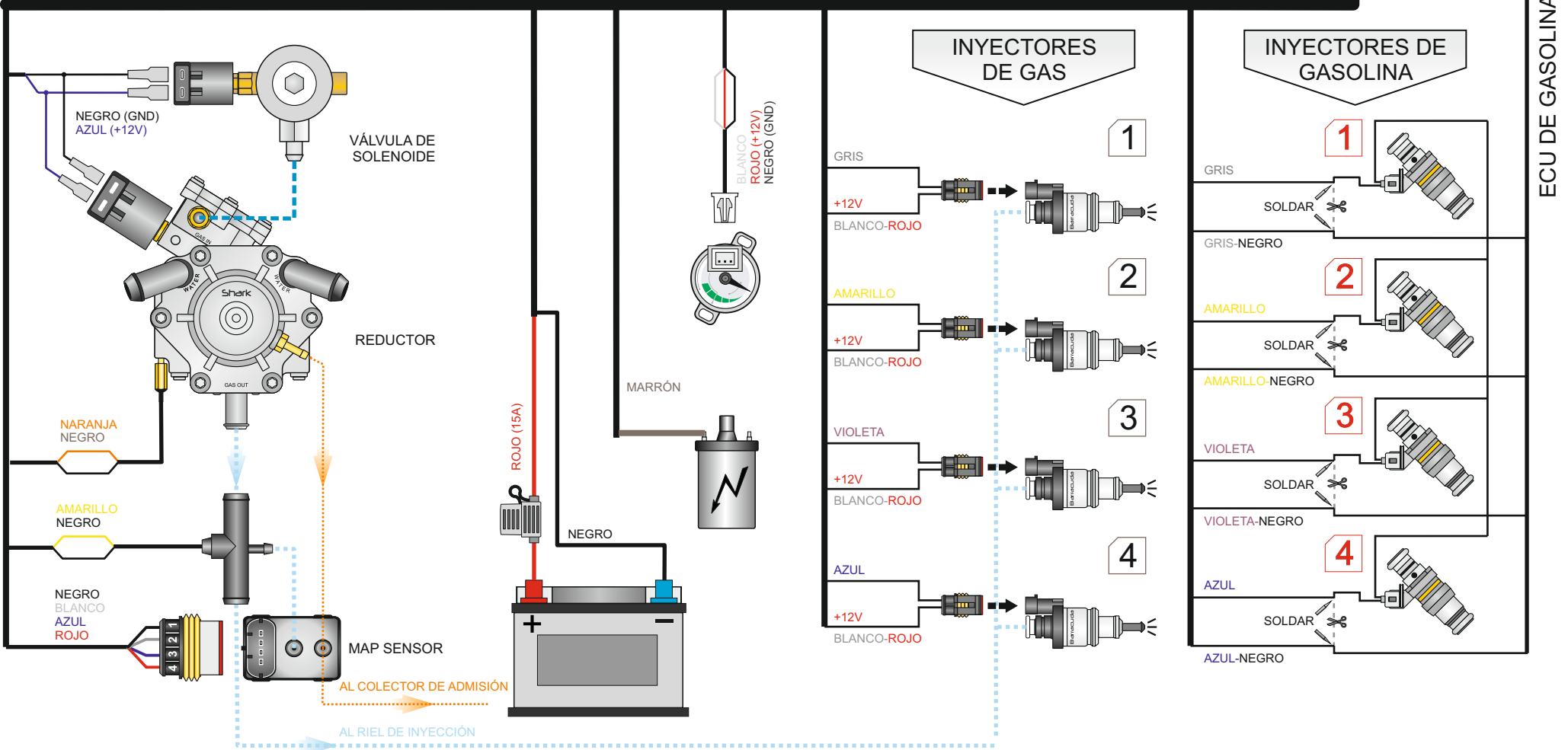
DIAGRAMA DE CONEXIÓN DE INSTALACIÓN DE GLP/GNC OPTIMA ECO-TEC
