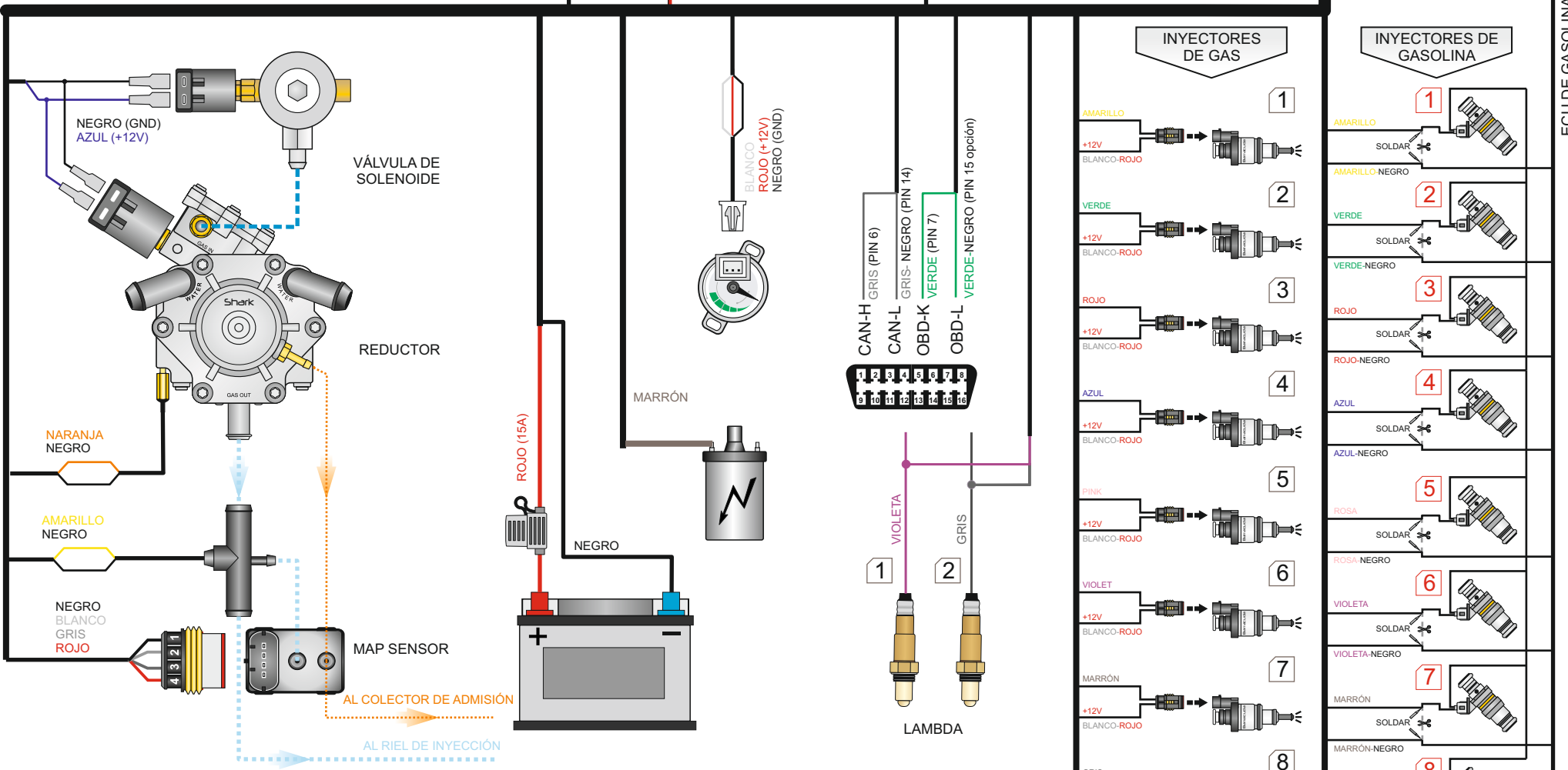
DIAGRAMA DE CONEXIÓN DE INSTALACIÓN DE GLP/GNC OPTIMA PRO-TEC
